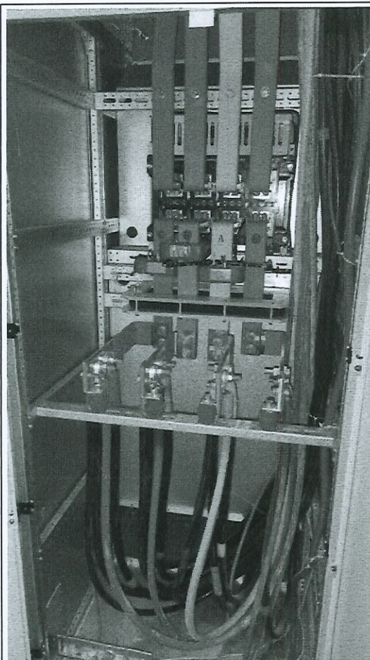
厂房2的800kVA出线柜
